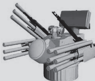
Зенитный автомат (ЗА)
