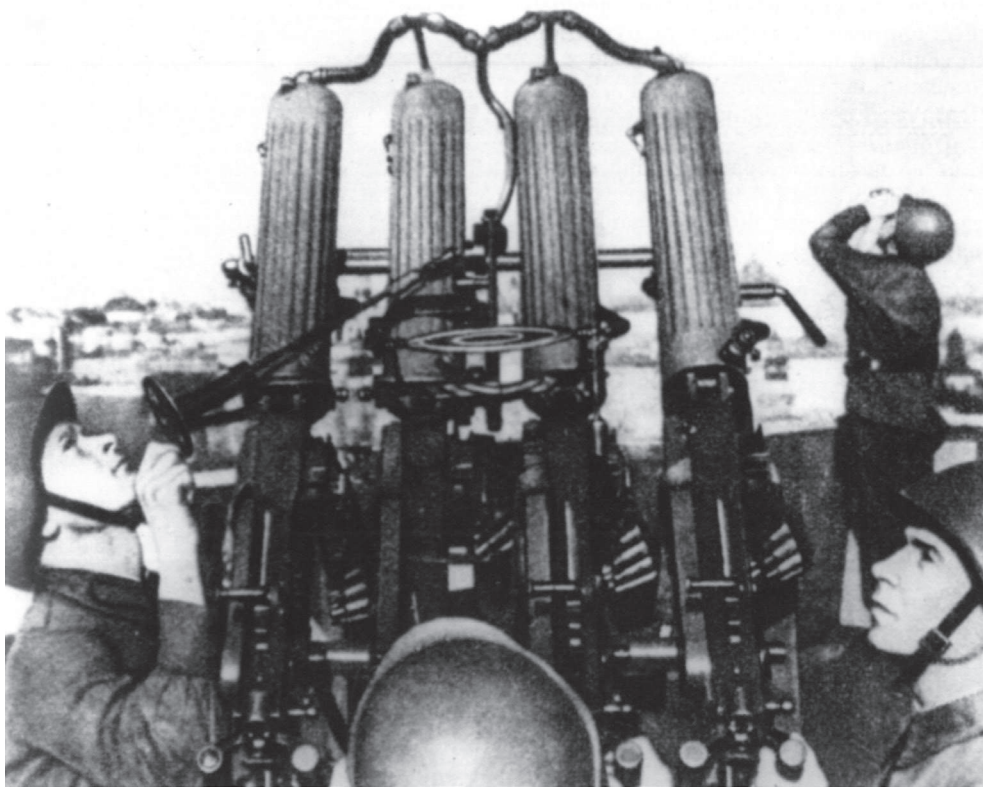
Счетверенная зенитная установка Н.Ф. Токарева под пулемет «Максим»
